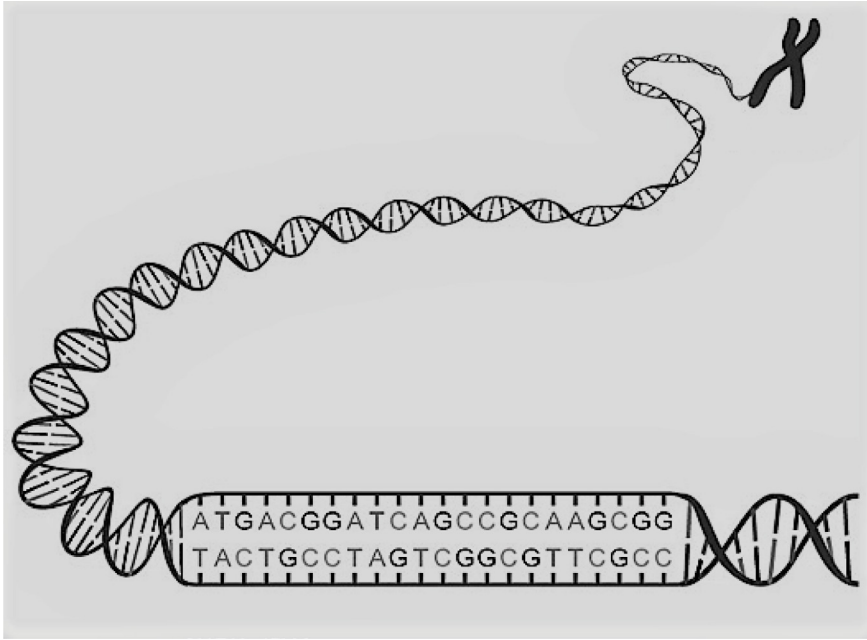
القواعد النيتروجينية في الـ DNA.
