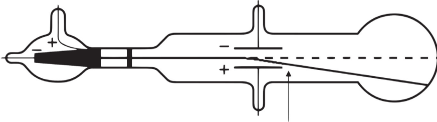
الشعاع منحرفاً نحو القطب الموجب
