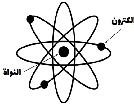
رسم تقريبي لبنية الذرة
